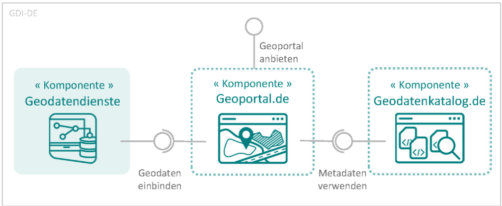
Abbildung 13: Komponentendiagramm Geoportal.de
