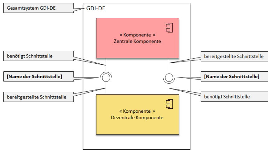
Abbildung 10: Beziehungen zwischen einer zentralen und dezentralen Komponente
