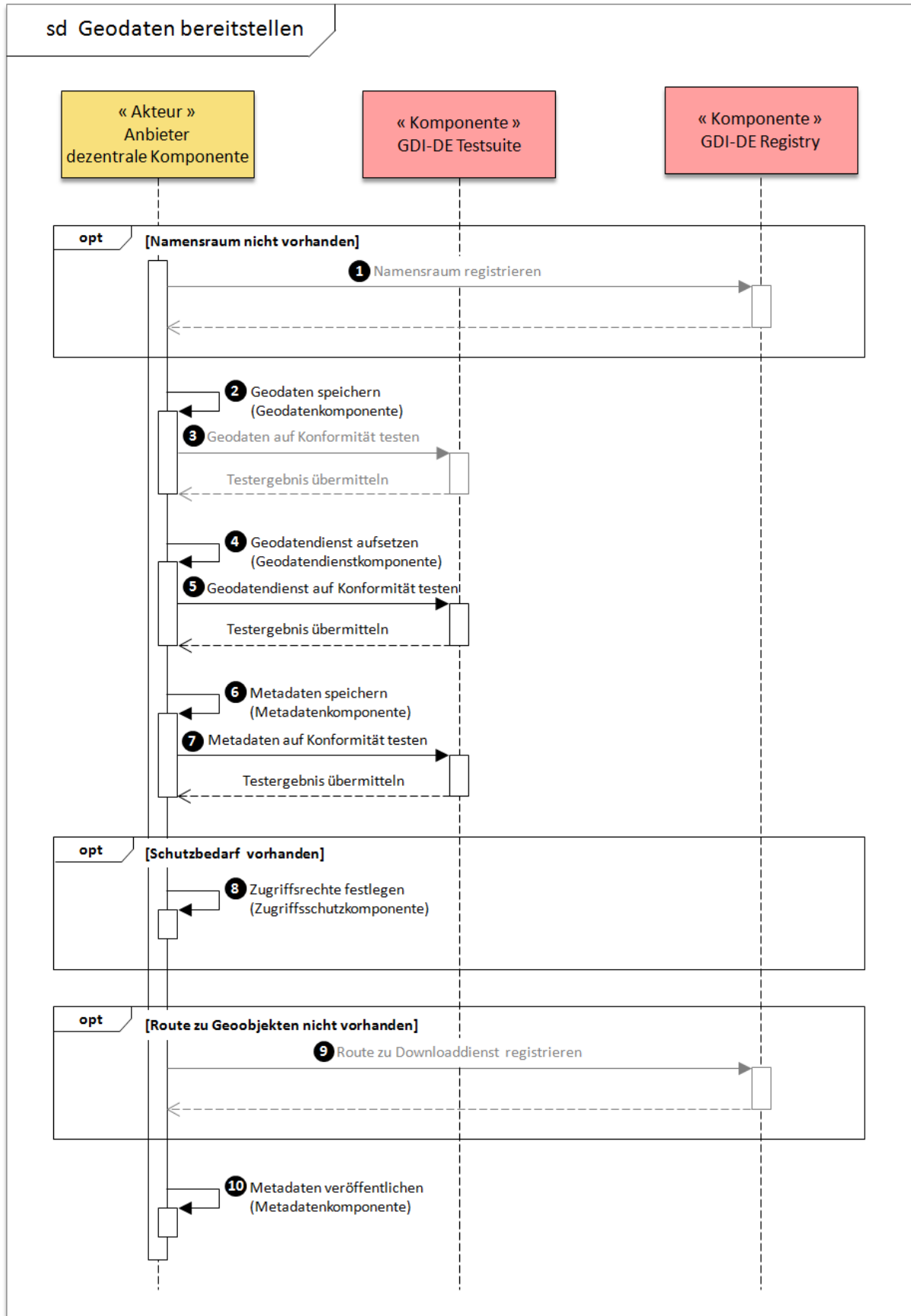
Abbildung 20: Sequenzdiagramm „Geodaten bereitstellen“
