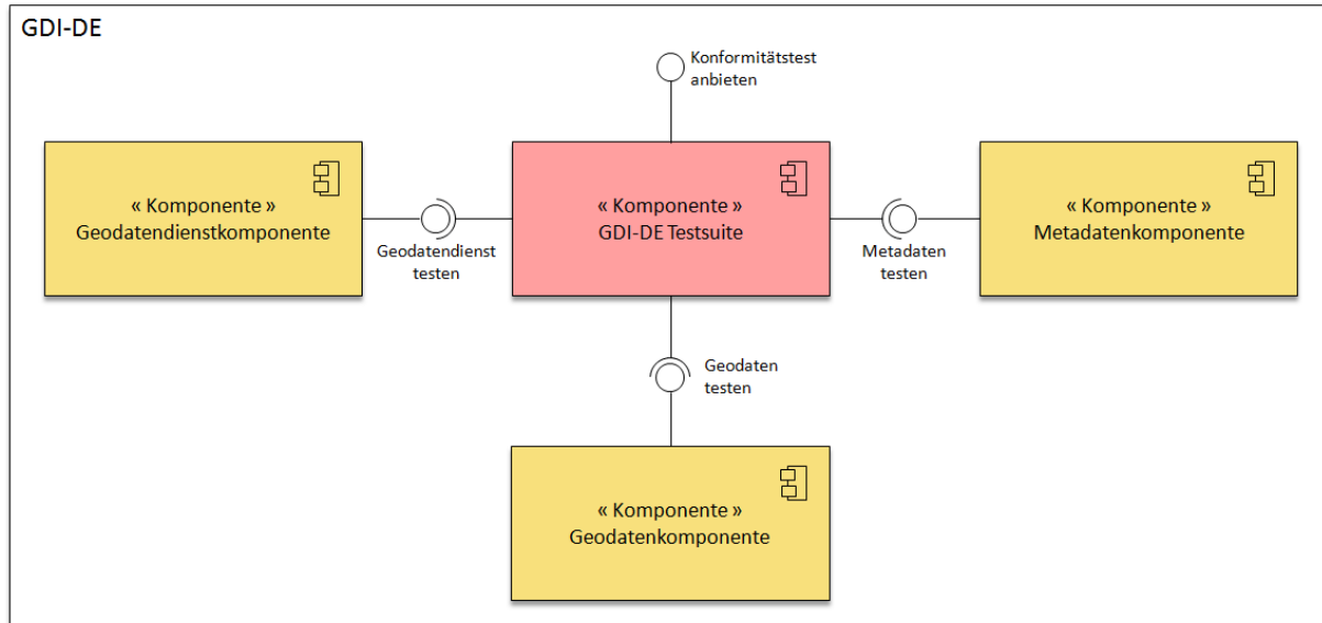
Abbildung 12: Komponentendiagramm GDI-DE Testsuite
