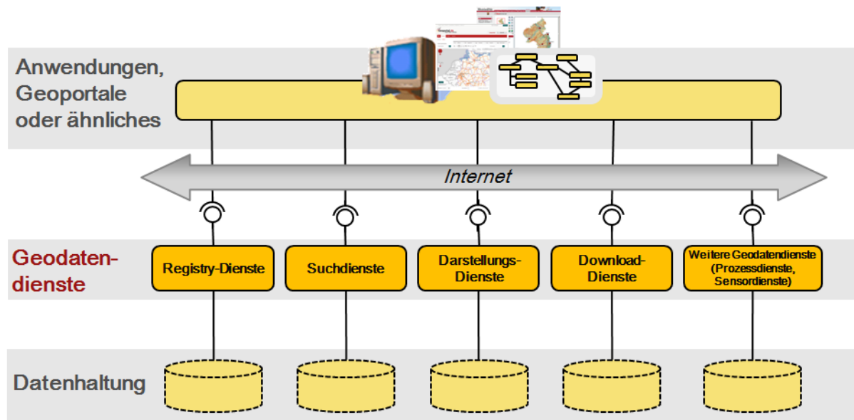
Abbildung 4: Schematische Darstellung der Architektur der GDI-DE
