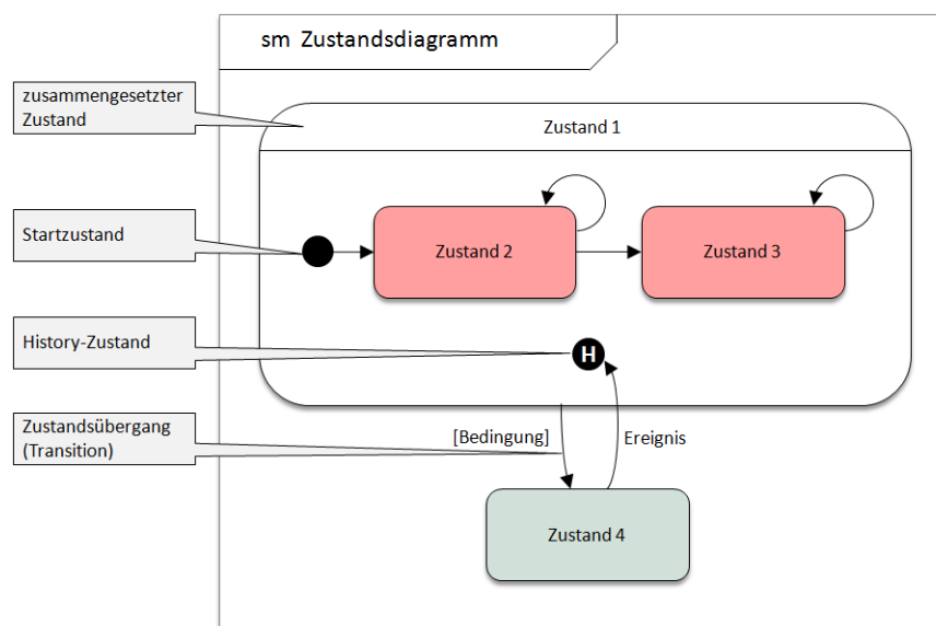
Abbildung 2: Notationselemente in einem Zustandsdiagramm
