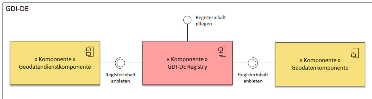
Abbildung 14: Komponentendiagramm GDI-DE Registry
