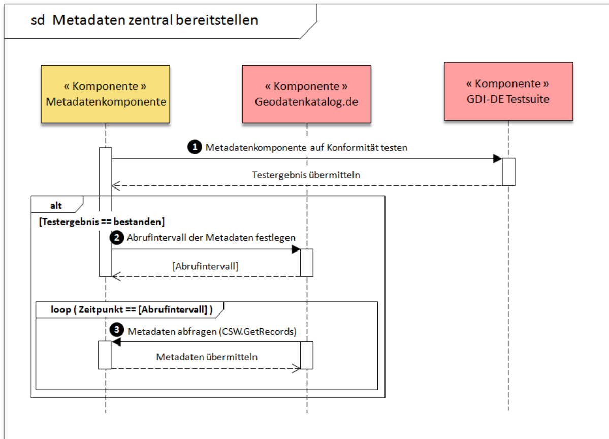
Abbildung 21: Sequenzdiagramm „Metadaten zentral bereitstellen“
