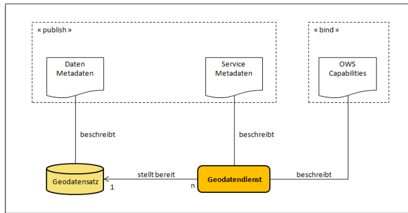
Abbildung 7: Geodaten und Geodatendienste mit Metadaten und Capabilities
