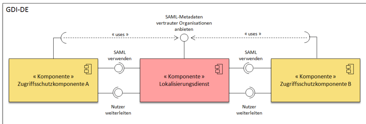
Abbildung 15: Komponentendiagramm Lokalisierungsdienst
