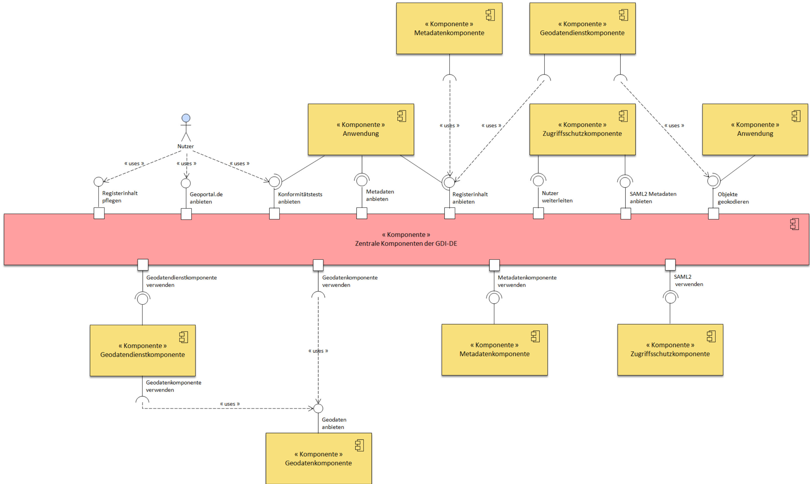
Abbildung 25: Architektur (Blackbox)
