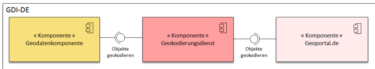
Abbildung 16: Komponentendiagramm Geokodierungsdienst
