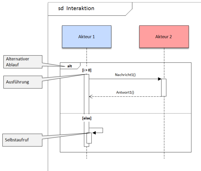
Abbildung 19: Notation zur Beschreibung von Interaktionen
