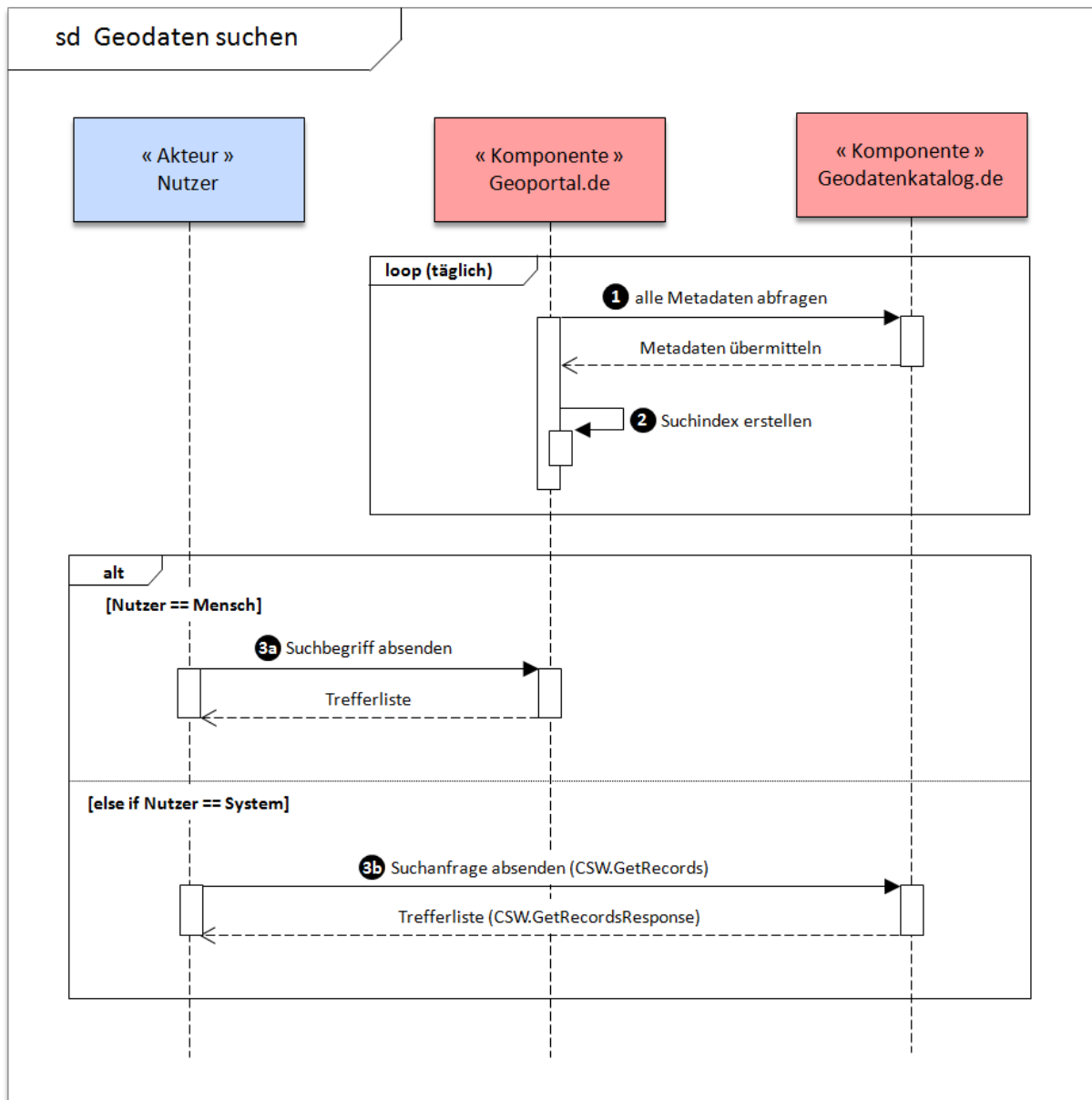
Abbildung 22: Sequenzdiagramm „Geodaten suchen“
