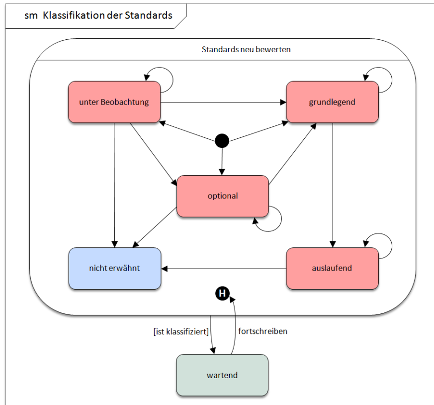
Abbildung 3: Klassifikation der Standards
