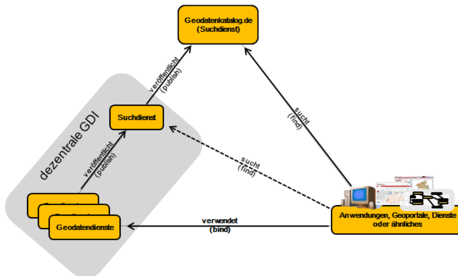
Abbildung 6: Publish-Find-Bind-Muster – übertragen auf die Architektur der GDI-DE
