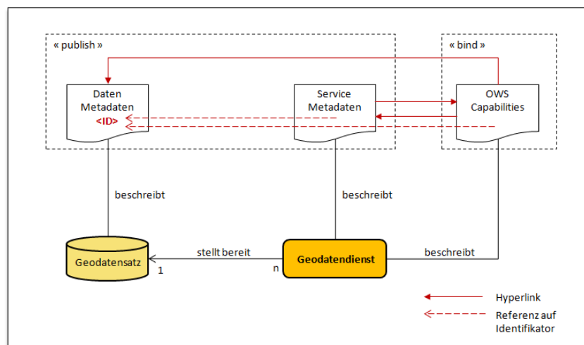
Abbildung 8: Kopplung der Geodaten und Geodatendienste
