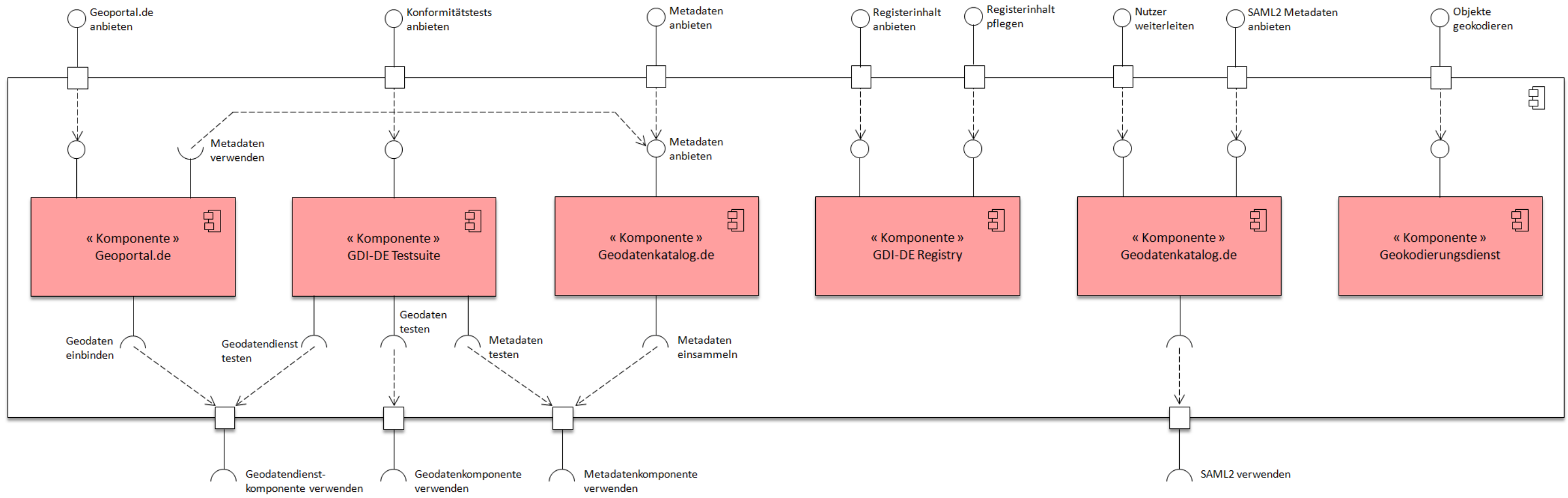
Abbildung 24: Architektur (Whitebox)
