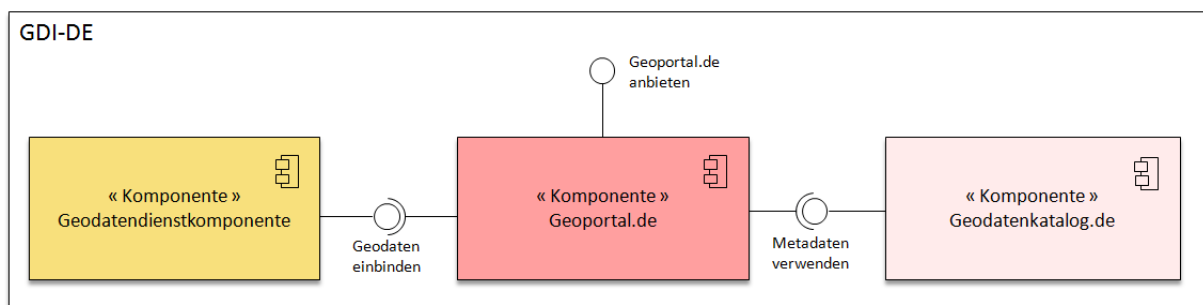
Abbildung 13: Komponentendiagramm Geoportal.de
