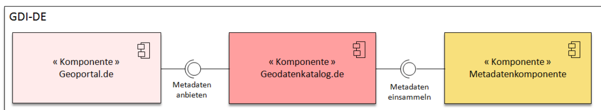
Abbildung 11: Komponentendiagramm Geodatenkatalog.de
