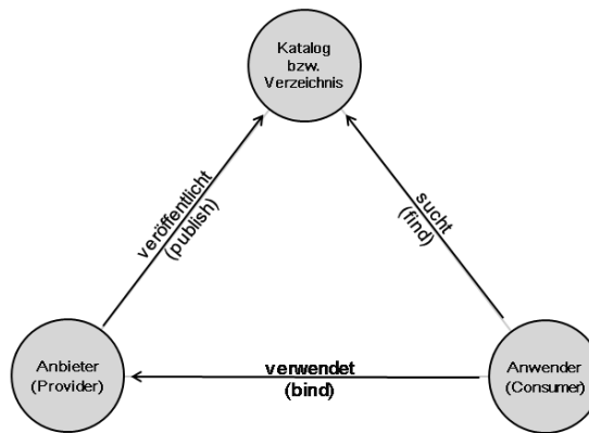
Abbildung 5: Allgemeines Publish-Find-Bind-Muster
