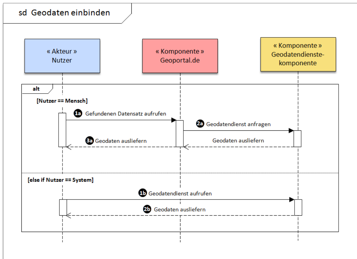
Abbildung 23: Sequenzdiagramm „Geodaten einbinden“
